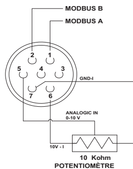
CONNECTEUR ENTRÉE/SORTIE
