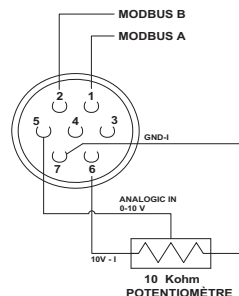
DÉTAIL CONNEXIONS
