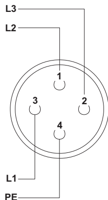
CONNECTEUR D'ALIMENTATION (TRIPHASÉ)
