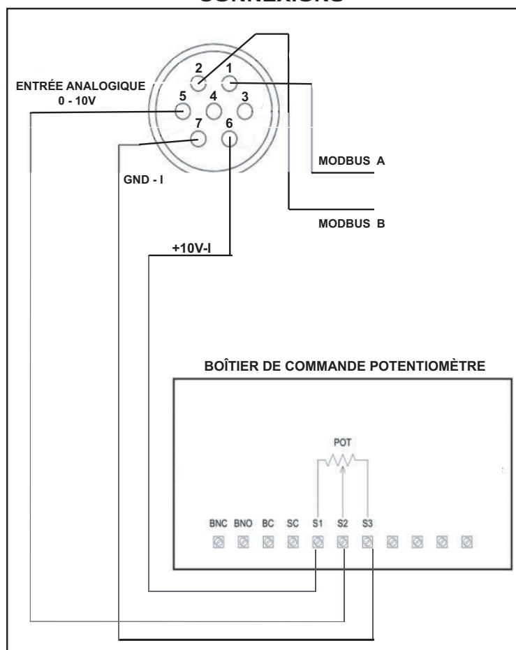
DÉTAIL CONNEXIONS
