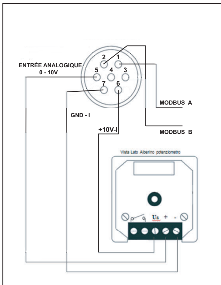
DÉTAIL CONNEXIONS
